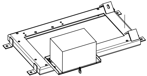
BATERIA IZQUIERDA
